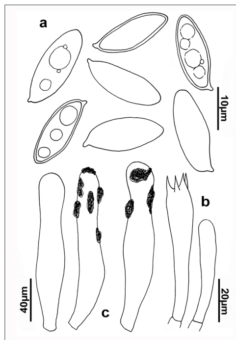
Gomphidius maculatus (Scop.) Fr., BAR2017102223, a. Basiidiósporas, b. Basidios, c. Cistidios.
