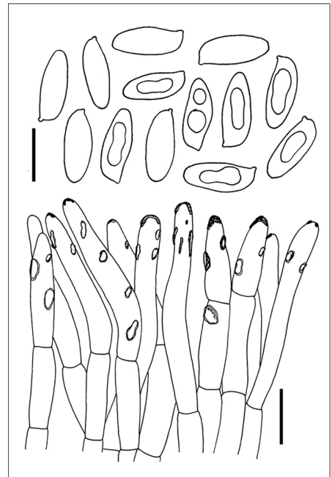
Rheubarbariboletus armeniacus (Quél.) Vizzini, Simonini & Gelardi, BAR2005090920, a. Basidiósporas, b. Pileipellis. Escala barra: a = 10 μ m, b. 20 μ m.
